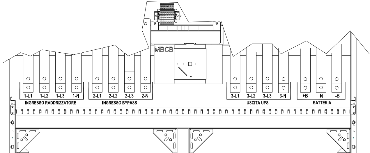
Figura 7 – Morsettiera KEOR HPE 400-500 kVA
