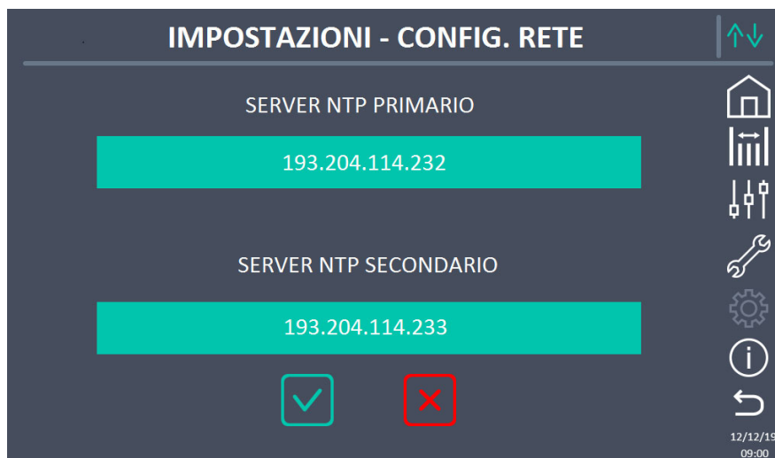
Figura 29 – Impostazione parametri NTP
