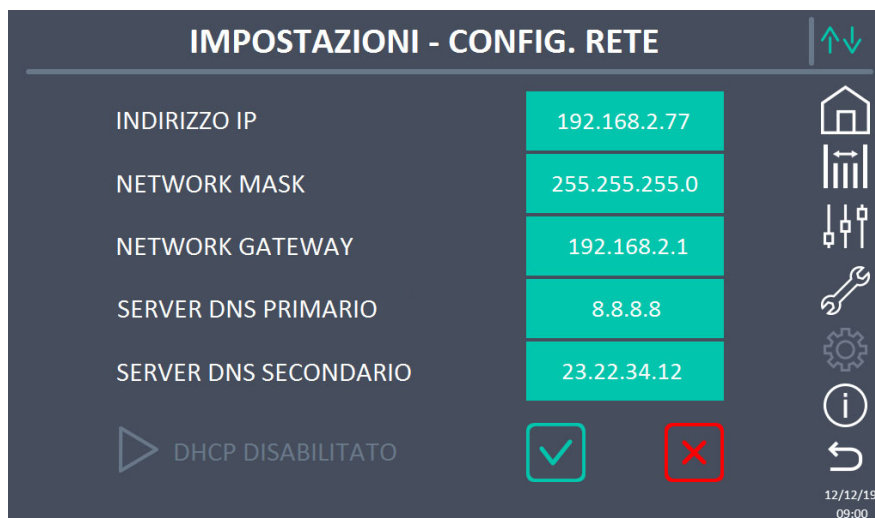
Figura 28 – Impostazione parametri LAN
