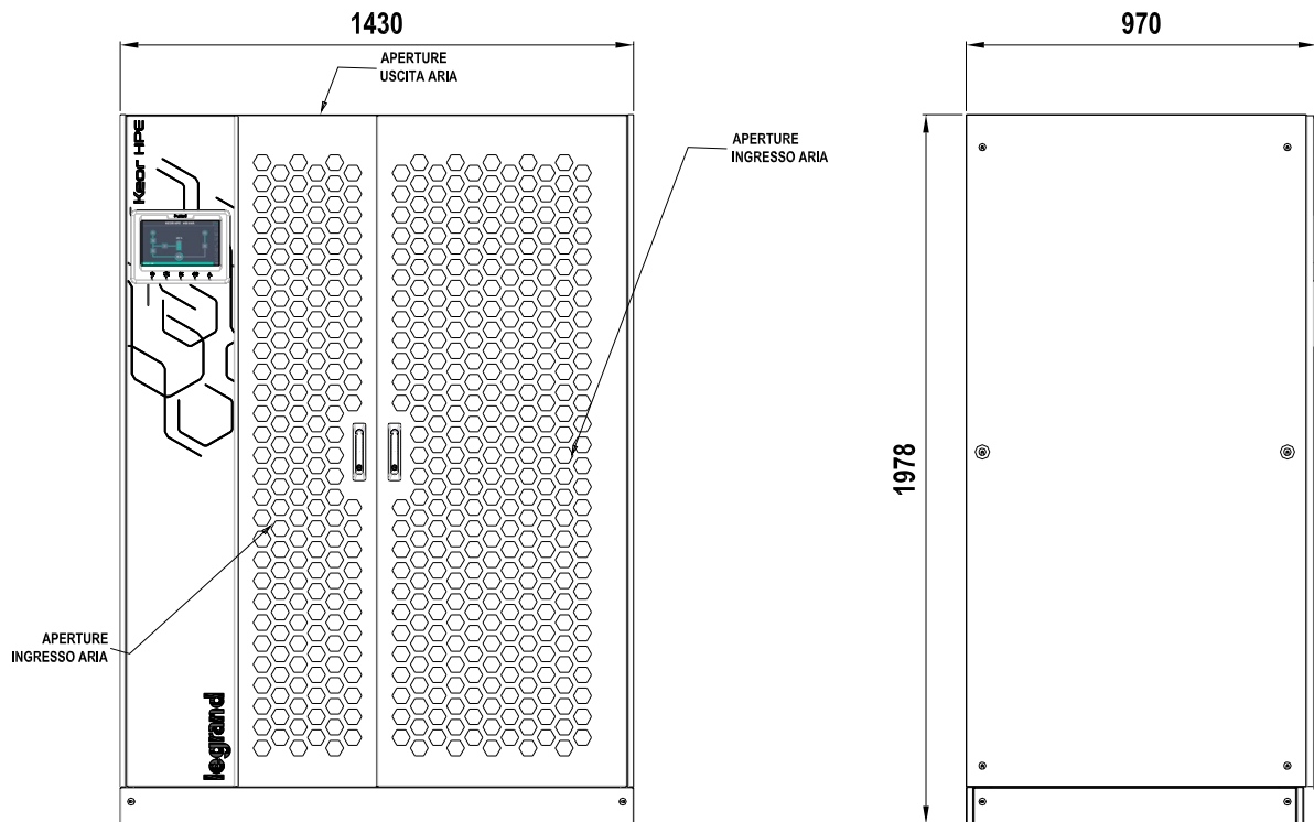
Figura 4 – Dimensioni di ingombro KEOR HPE 400-500kVA
