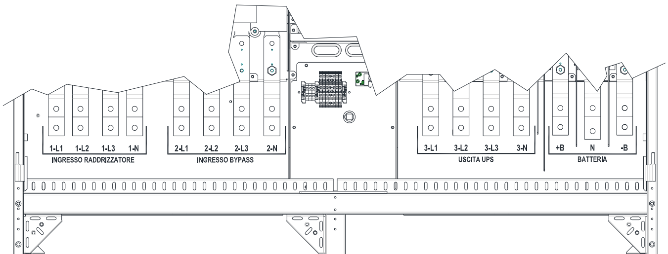
Figura 7A – Morsettiera KEOR HPE 600 kVA
