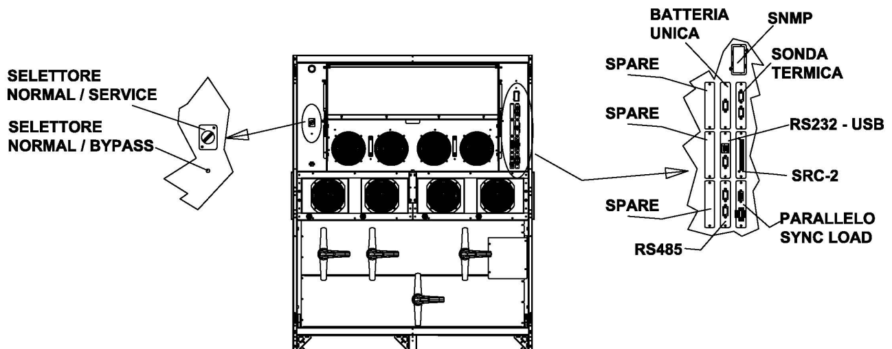
Figura 9A – Posizione schede di interfaccia KEOR HPE 600kVA
