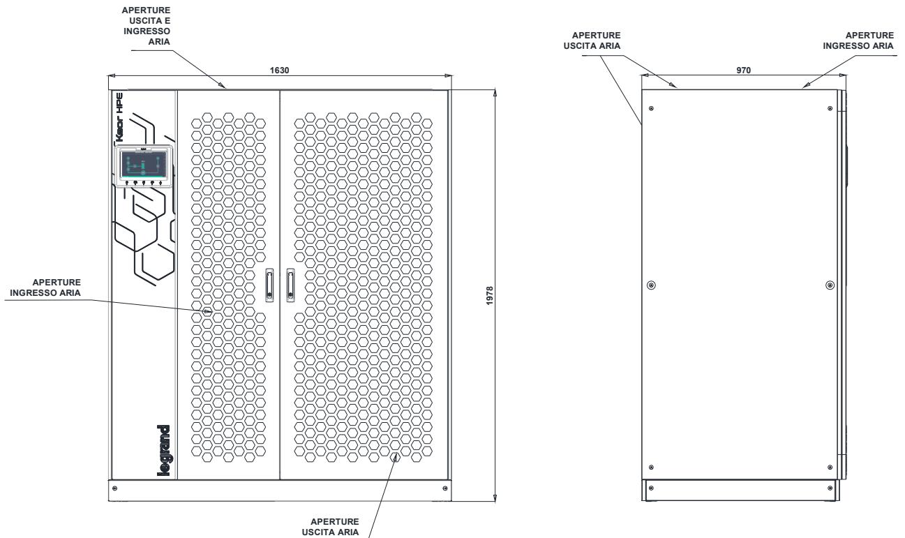
Figura 4A – Dimensioni di ingombro KEOR HPE 600kVA
