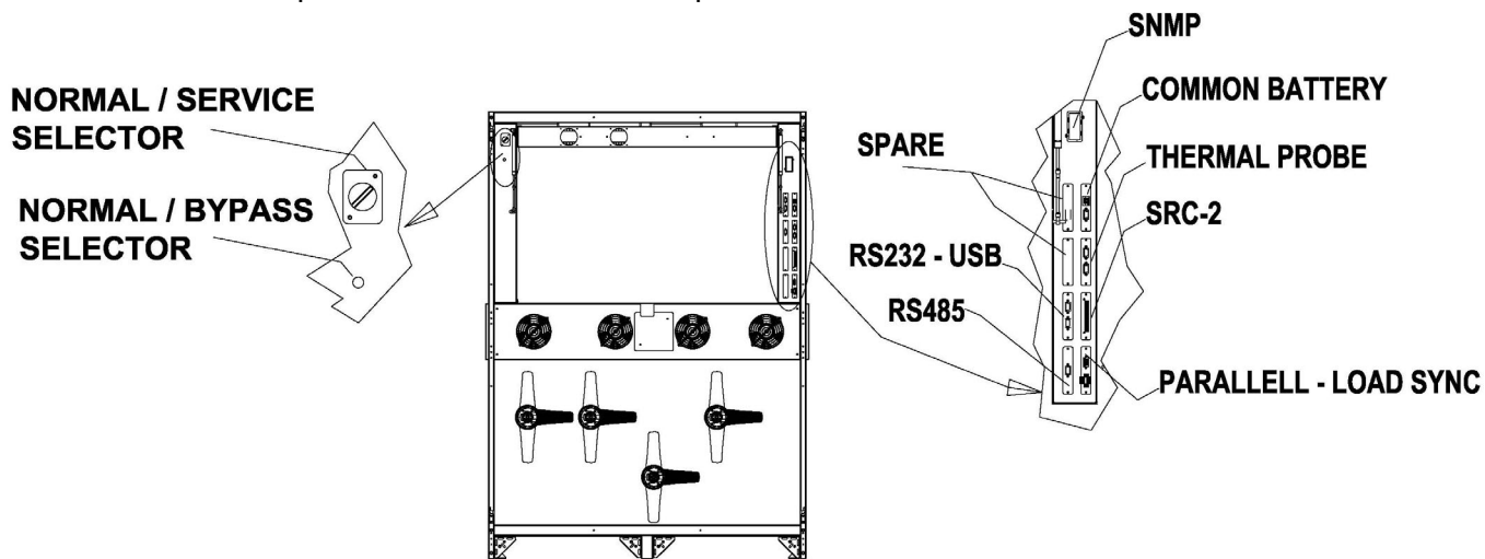
Illustration 9 – Position des interfaces de série du KEORHPE 400-500 kVA
