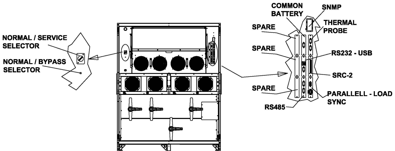
Illustration 9A – Position des interfaces de série du KEORHPE 600 kVA
