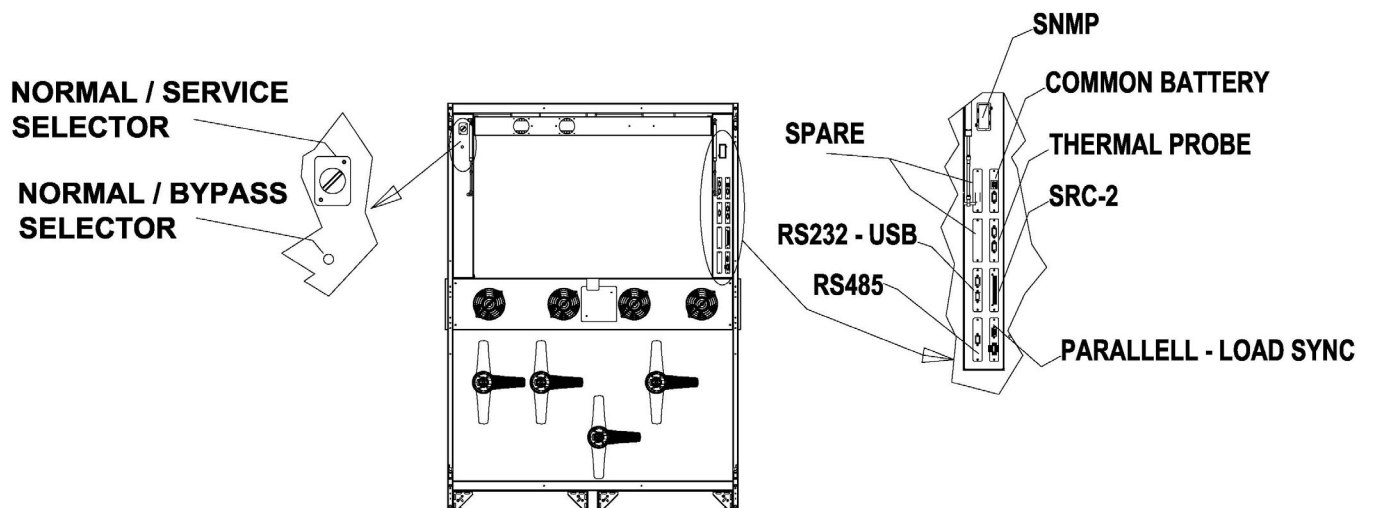
Figura 9 – Posizione schede di interfaccia KEOR HPE 400-500kVA
