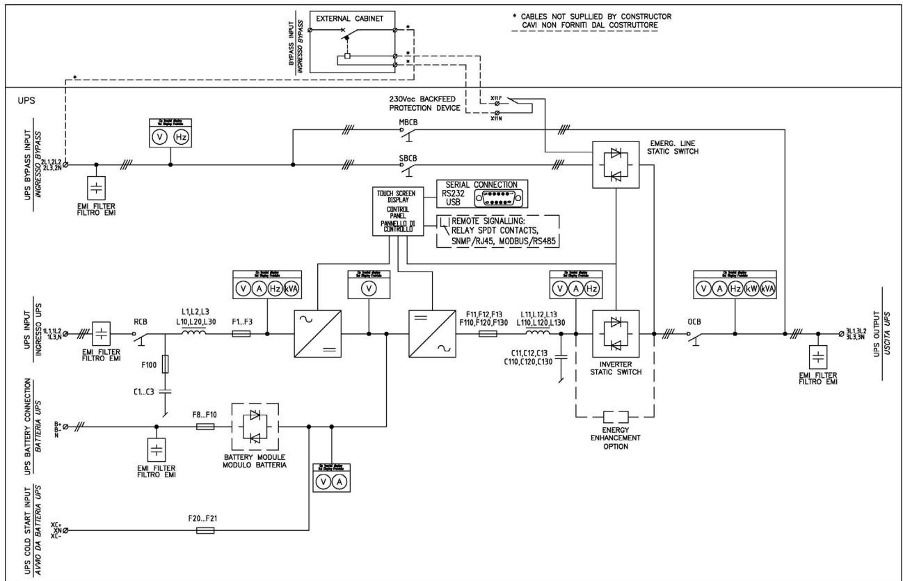
Illustration 6 – Diagramme à une ligne KEOR HPE 400-500-600 kVA avec connexion à un périphérique externe
