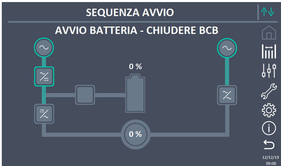
Figura 15 – Avvio batteria
