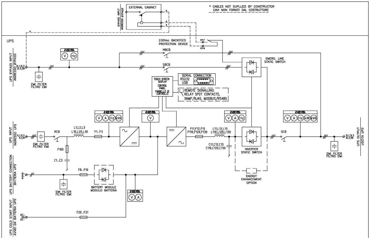
Figura 6 – Schema unifilare KEOR HPE 400-500-600 kVA con collegamento al dispositivo esterno
